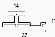
Aluminum clip AF609
