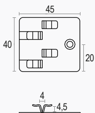
Edelstahl-Doppelnutzungsclip für Classic Verkleidung AF611
