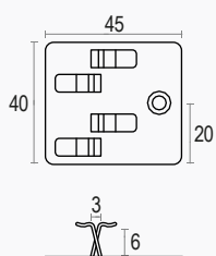
Clip AF607 für Classic Bodenbelag Doppelnutzung
