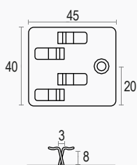
Clip AF608 für Professional Bodenbelag Doppelnutzung
