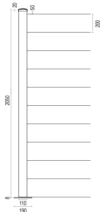
H 2050 n° 10 slats
