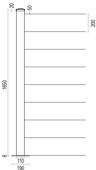
H 1650 n° 8 slats
