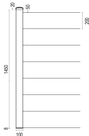
H 1450 n° 7 slats
