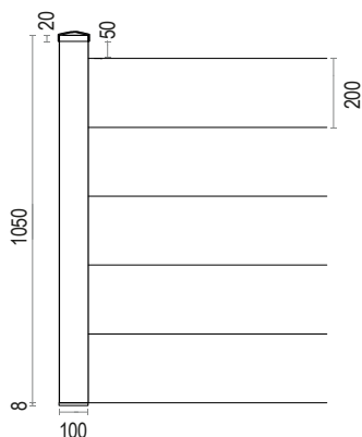
H 1050 n° 5 slats
