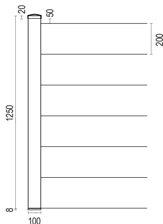
H 1250 n° 6 slats
