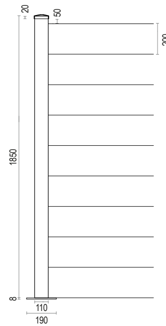
H 1850 n° 9 slats
