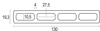
"Vedo non vedo" slat
