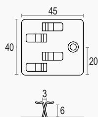
Clip AF607 per pavimento Classic doppio uso
