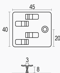
Clip AF608 per pavimento Professional doppio uso
